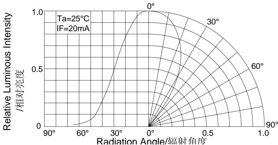
DIRECTIVITY/指向特性
